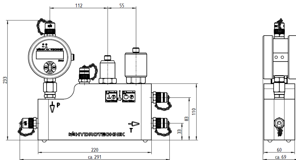
Abbildung 1: Technische Zeichnung CX 197
